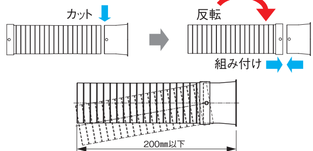
※ 排水勾配(5°以下)に対応した取付方法
