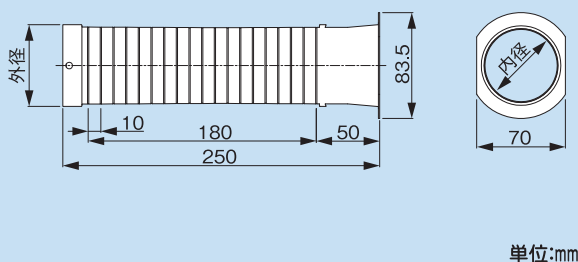
寸法図
