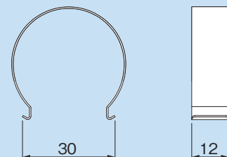
寸法図
