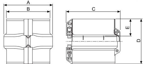
寸法図
